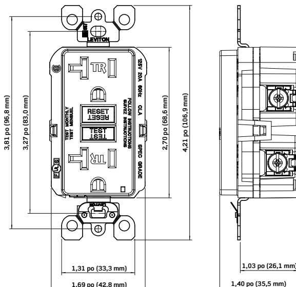
Prise à DDFT SmartlockPro MD avec fonctions d'autovérification de 20A
