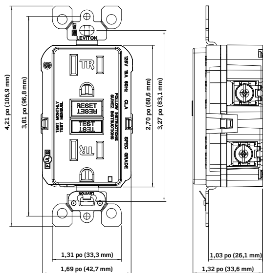
Prise à DDFT SmartlockPro MD avec fonctions d'autovérification de 15A
