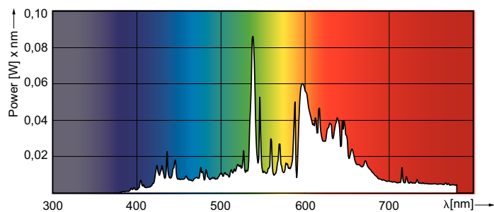
CDM-R Elite 35W /930 PAR20 E27
